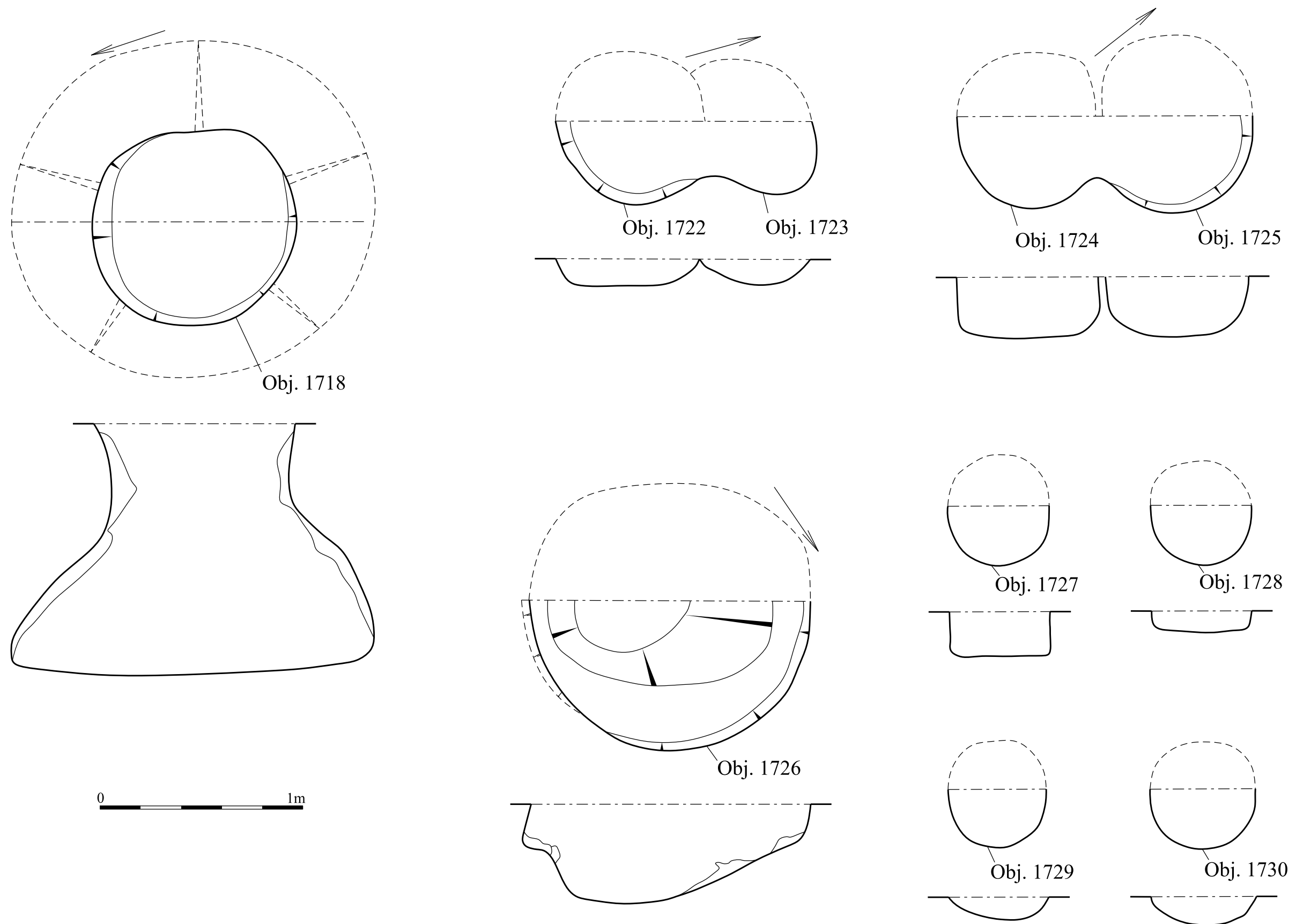
Obr. 6. Polešovice 2013 - kresebný plán objektu 1718, 1722-1730
