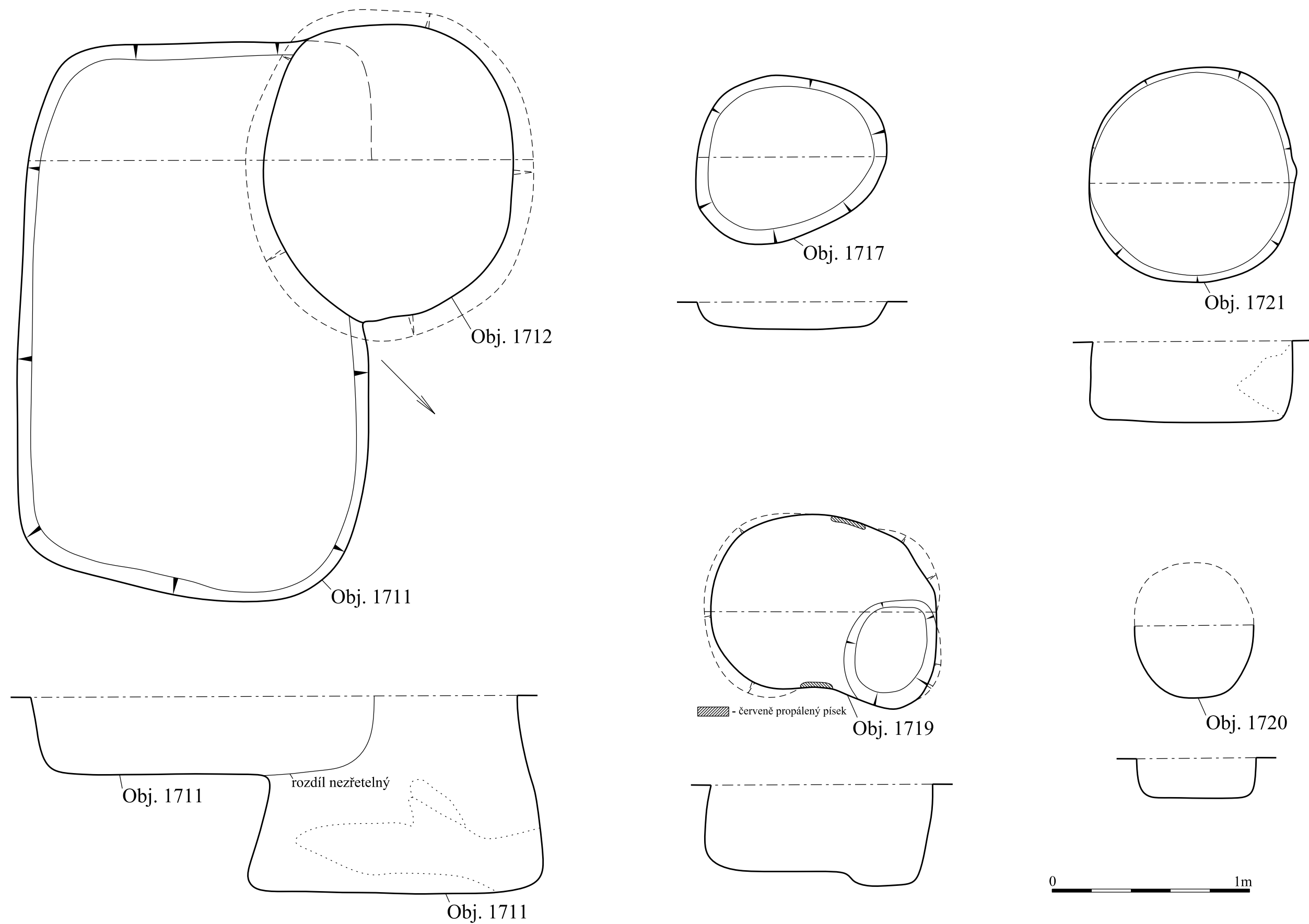
Obr. 5. Polešovice 2013 - kresebný plán objektu 1711, 1712, 1717, 1719, 1720, 1721
